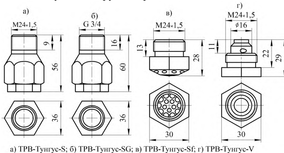
Рисунок 9 – Насадки-распылители
