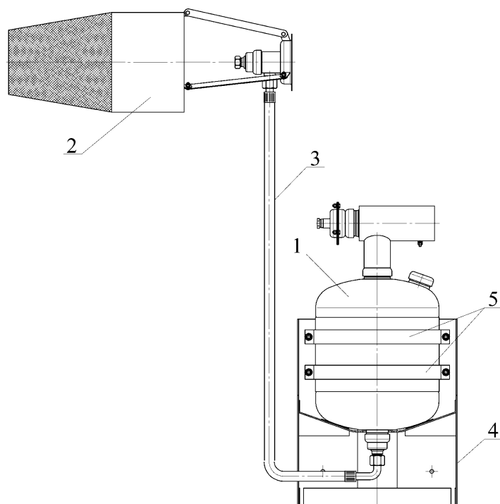
Рисунок 10 – МППВК с горизонтальным расположением эжектора 1-МППВК; 2-пеногенератор; 3-трубопровод; 4-стапель; 5-хомуты
