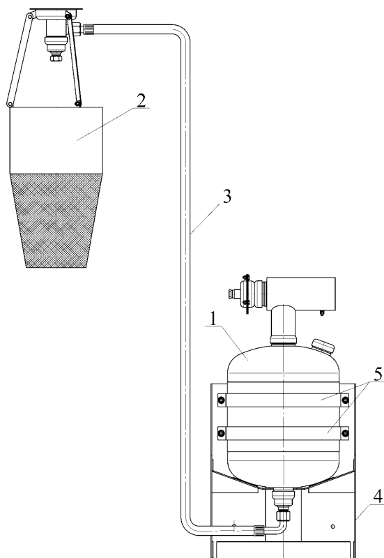
Рисунок 9 – МППВК с вертикальным расположением эжектора 1-МППВК; 2-пеногенератор; 3-трубопровод; 4-стапель; 5-хомуты
