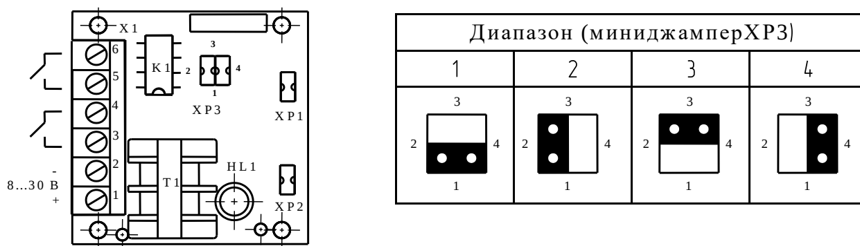
Рисунок 1 – Настройка чувствительности
